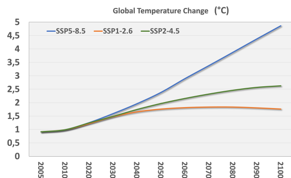
Globale Temperaturzunahme gegenüber vorindustrieller Zeit. Schematische Darstellung.
