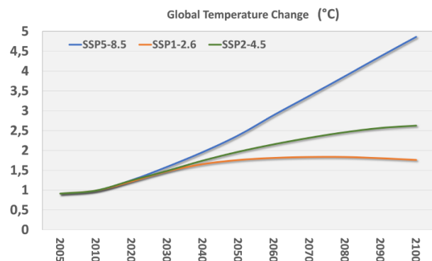
Globale Temperaturzunahme gegenüber vorindustrieller Zeit. Schematische Darstellung.
